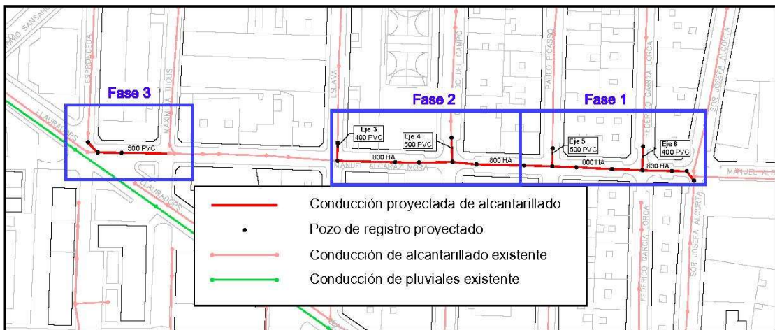
Red de alcantarillado proyectada
